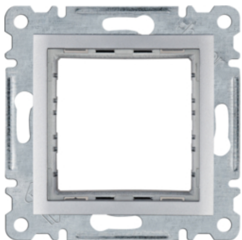
Adaptér pro přístroje 45x45 mm, stříbrná mat
